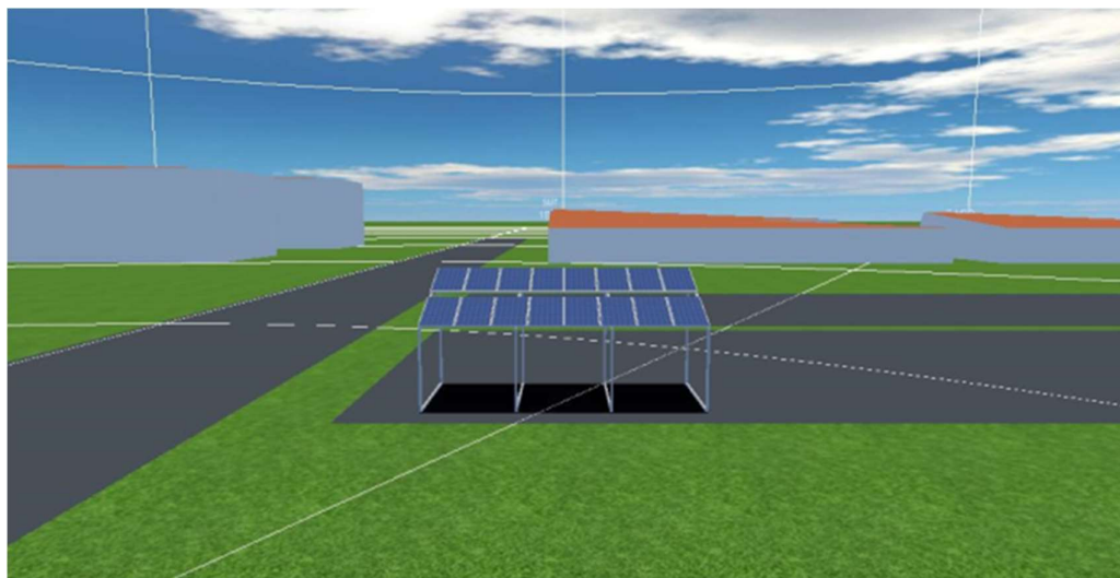
Figura 40. Visualização do sistema em 3D, gerada pelo PVSol
