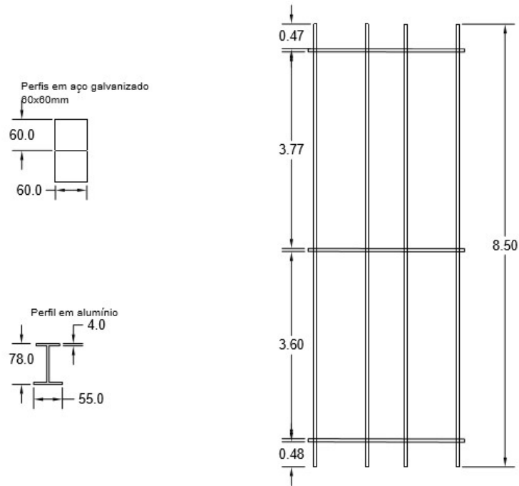
Figura 19. Ilustração com vista superior da estrutura de sustentação
