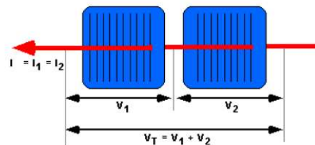
Figura 24. Exemplo de ligação de módulos fotovoltaicos em série.
