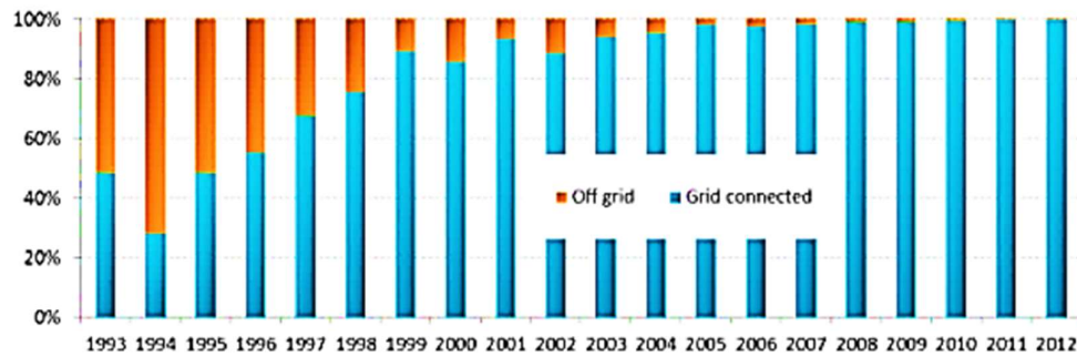
Figura 9. Evolução dos sistemas fotovoltaicos off grid e on grid .
