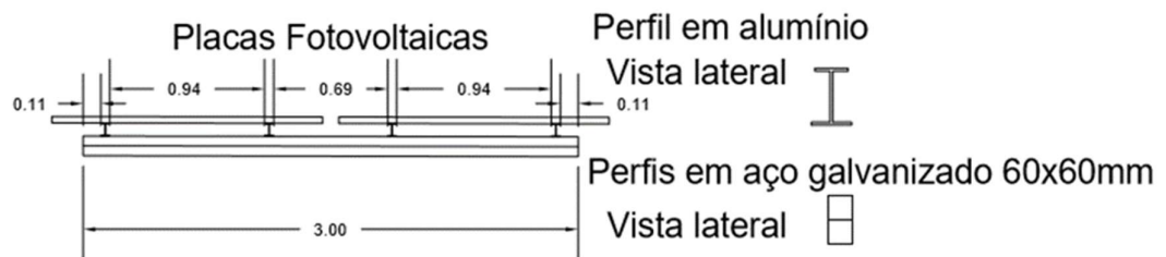
Figura 20. Ilustração com vista lateral da estrutura de sustentação
