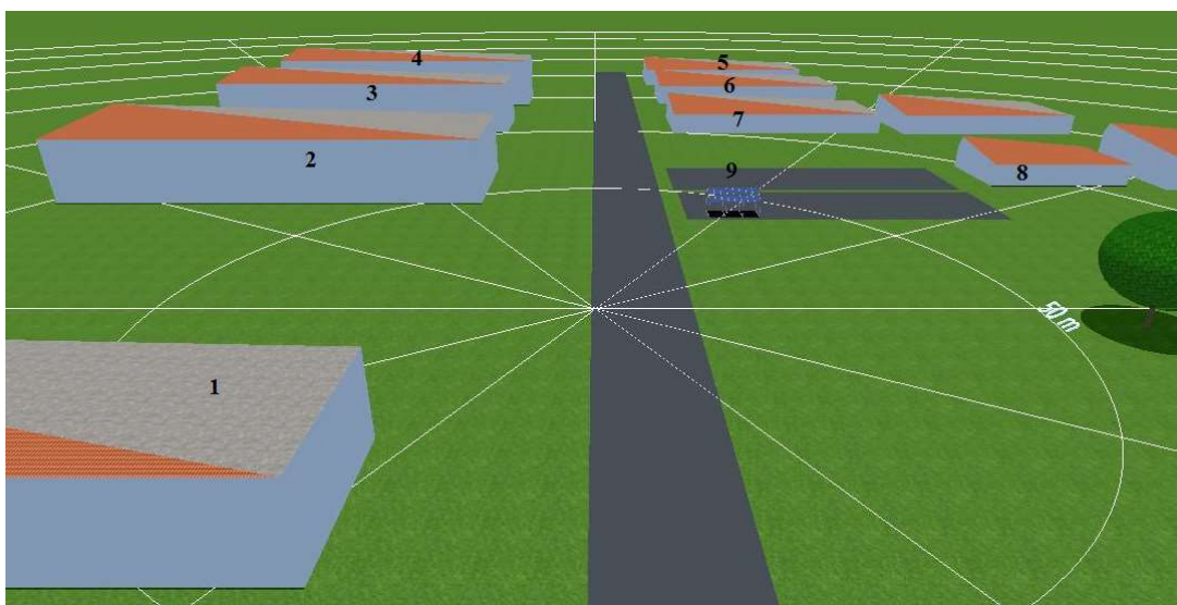
Figura 39. Disposição do sistema, prédios e árvore nas proximidades, gerada pelo PVSol
