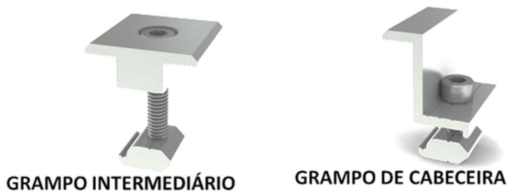
Figura 22. Grampos de fixação intermediária e final para painéis fotovoltaicos
