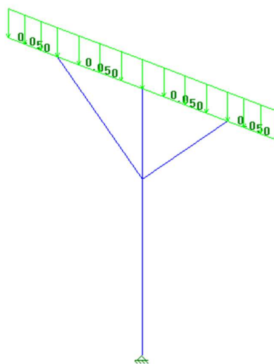
Figura 56. Carregamento na estrutura devido ao peso das placas – (kgf/m 2 )
