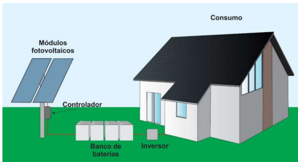
Figura 10. Esquematização de um sistema isolado (Off-Grid).
