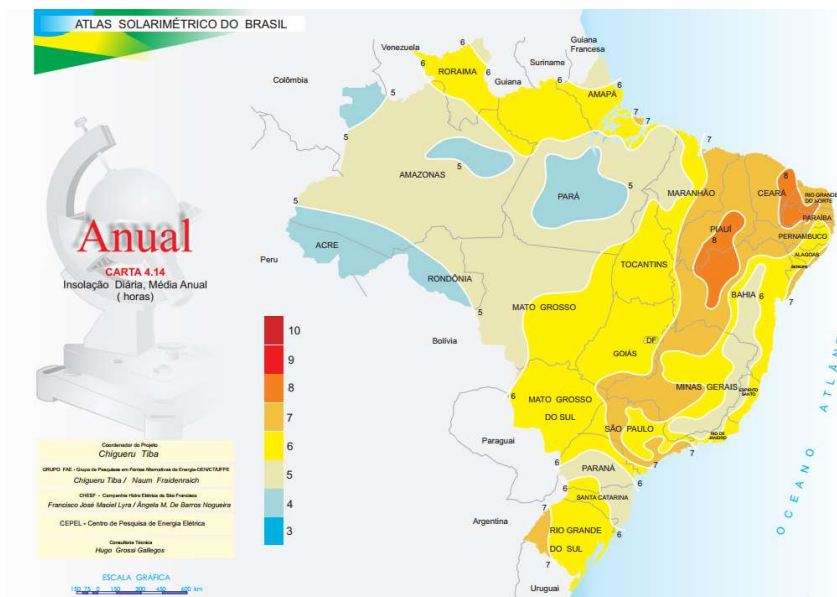
Figura 33. Média anual da insolação diária em horas do Brasil
