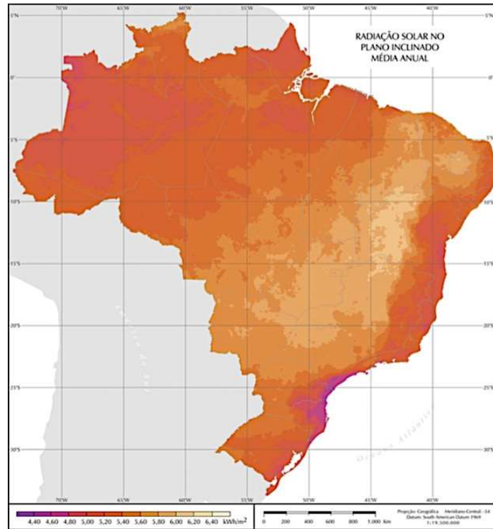
Figura 3. Mapa do potencial energético solar brasileiro de radiação solar no plano inclinado média anual
