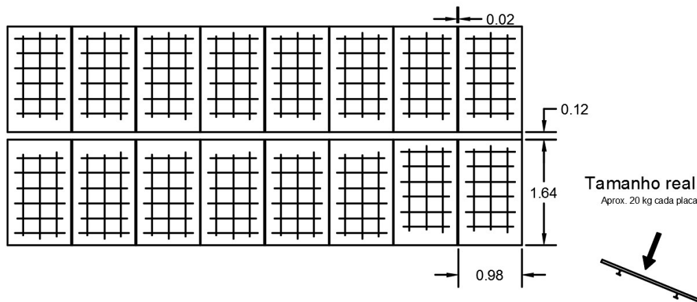
Figura 21. Vista Superior das Placas Fotovoltaicas
