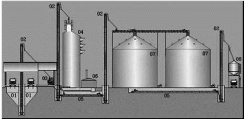
Figura 2: fluxo de grãos dentro de uma unidade armazenadora.
